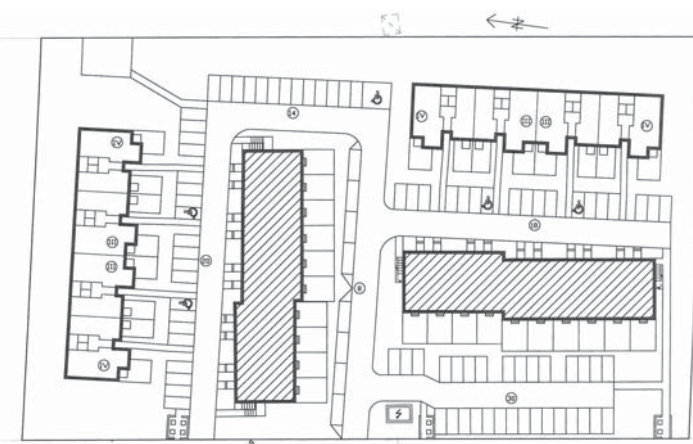
OSIEDLE REJTANA W JÓZEFOWIE - ZAGOSPODAROWANIE TERENU 1:500 ARCH. JAN PALLADO
